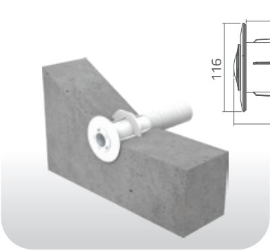
Conduits
