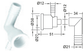
L-Type Jet Body
