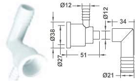
L-Type Jet Body
