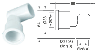
L-Type Jet Body
